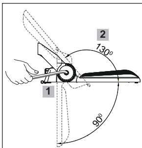
Angle adjustment تنظیم زاویه
